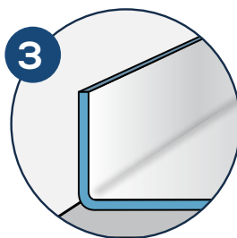
3 Dra upp insulParq 2+ längs väggarna
